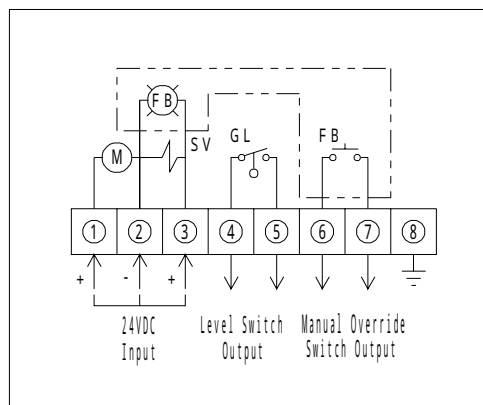
フィードボタン有り
