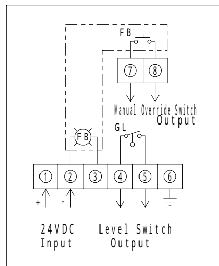
フィードボタン有り
