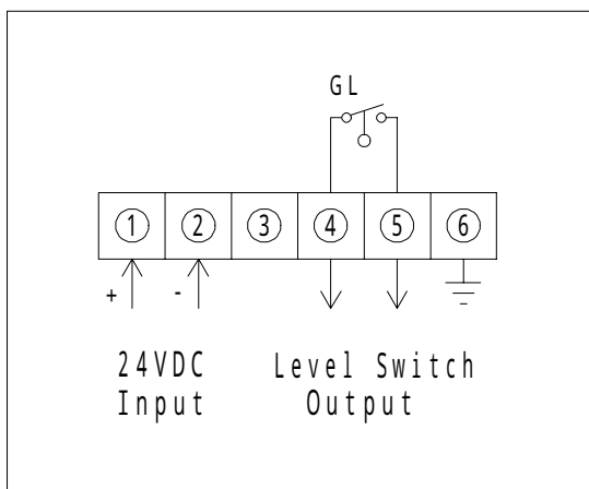
フィードボタン無し
